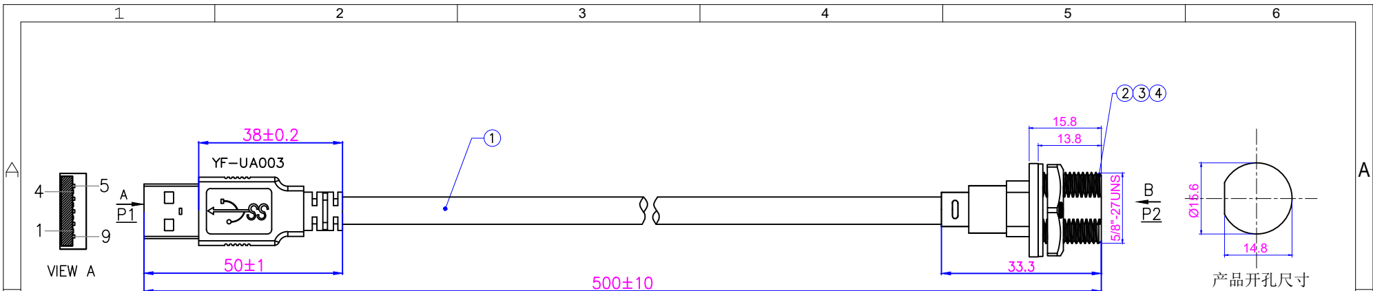
USB3.0 A/M 短体
