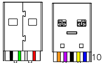
4 3 2 1 9 8 7 6 5 USB3.0 公头焊接面
