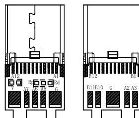
TYPE C3.0 母头焊接面
